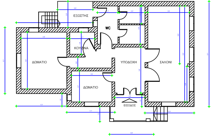
ΚΑΤΟΨΗ ΙΣΟΓΕΙΟΥ
