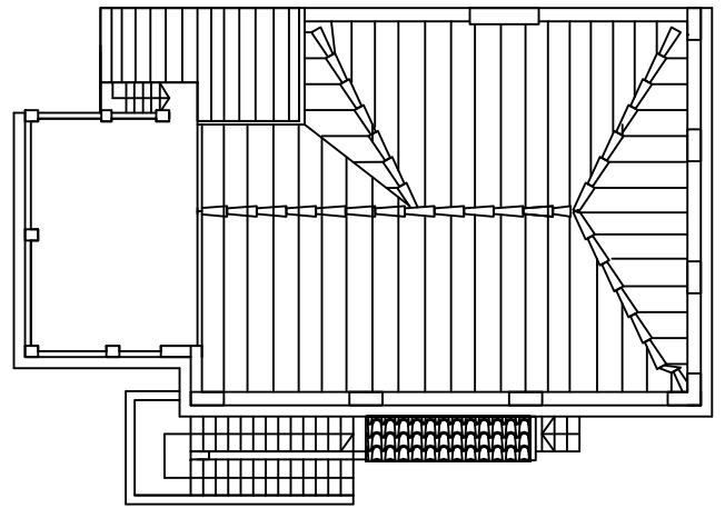
ΚΑΤΟΨΗ ΣΤΕΓΗΣ ΚΑΙ ΒΑΤΟΥ ΔΩΜΑΤΟΣ
