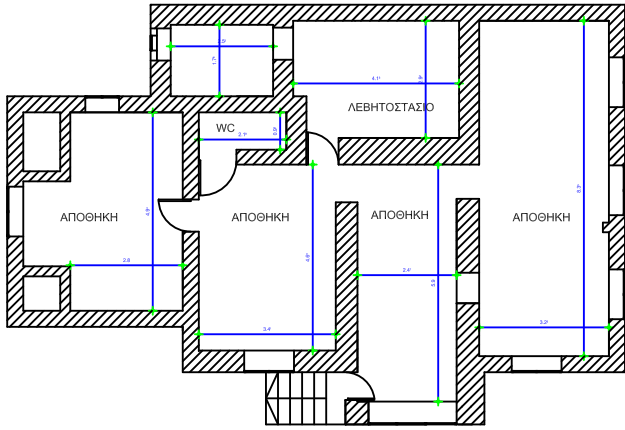
ΚΑΤΟΨΗ ΥΠΟΓΕΙΟΥ
