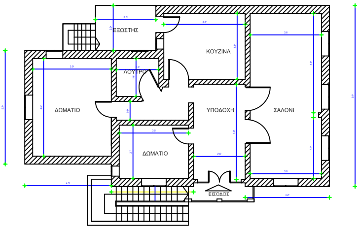
ΚΑΤΟΨΗ ΠΡΩΤΟΥ ΟΡΟΦΟΥ
